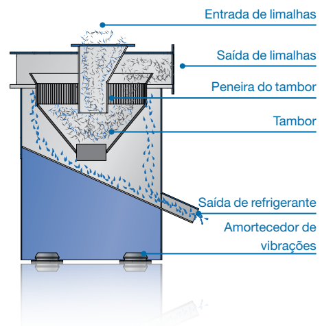
Esquema de princípio do modelo VSZ
