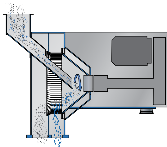
Esquema de princípio do modelo HSZ
